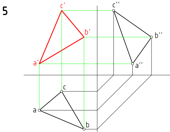
Hallar la proyección vertical del triángulo ABC.
