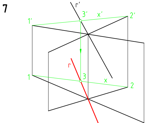
Hallar la proyección horizontal de la recta R coplanaria con las demás.
