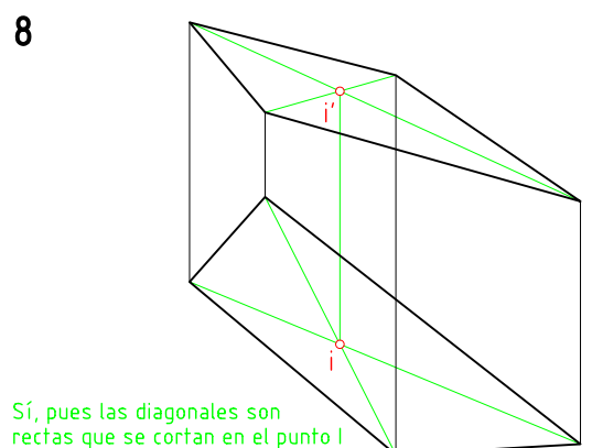
Comprobar si los cuatro vértices del cuadrilátero son coplanarios.
