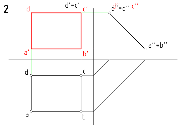
Hallar la proyección vertical del cuadrilátero ABCD.
