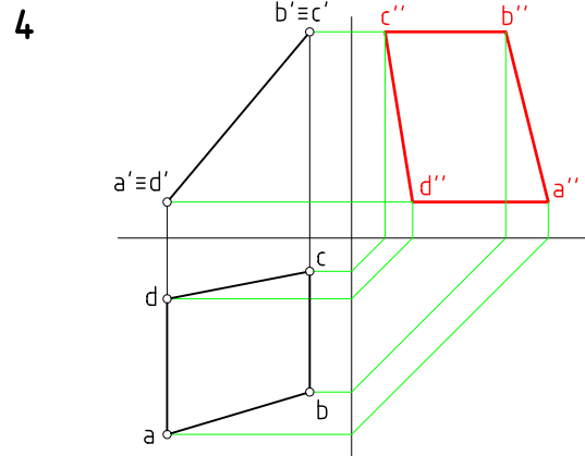
Hallar la proyección lateral del cuadrilátero ABCD.
