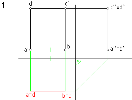
Hallar la proyección horizontal del cuadrilátero ABCD.
